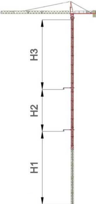
Secuencia de montaje
