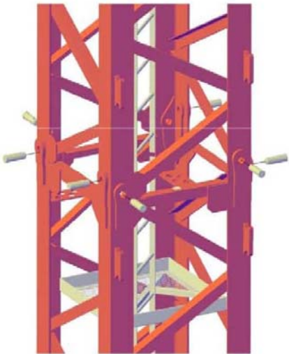
Sistema de Unión de los Tramos mediante bulones de Ø 50 x 170 mm
