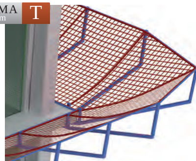
Red de seguridad sujeta a consolas para su utilización horizontal. Safety net tied to brackets for horizontal use.
