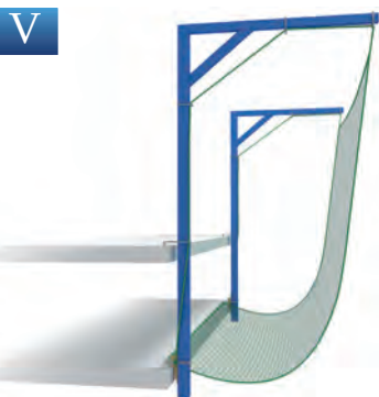
Red de seguridad con cuerda perimetral, para utilizar con horcas o pescantes. Safety net with border rope, attached to a gallows type support.
