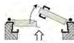
Sentido de apertura a derechas (DX)
