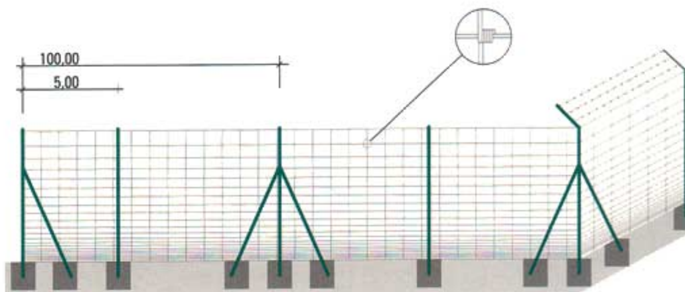
ALZADO, TIPO DE CERRAMIENTO
