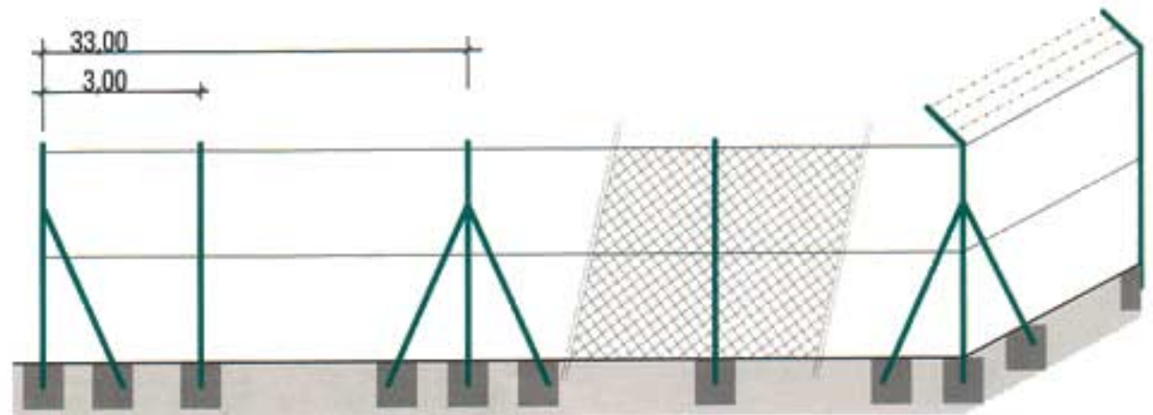
ALZADO TIPO DE CERRAMIENTO
