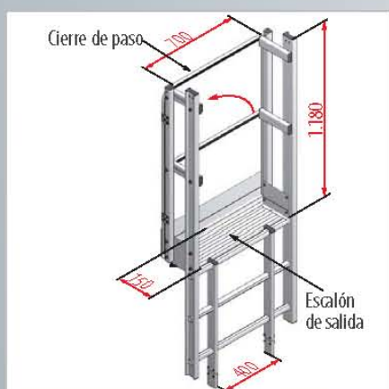
Salida ancha con gradilla
