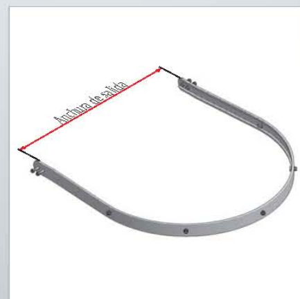
Anillo de protección dorsal para salida
