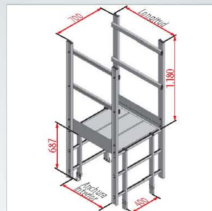
Salida ancha con puente
