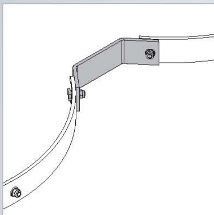
Conexión para anillo doble
