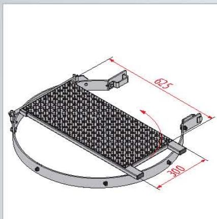
Plataforma intermedia abatible
