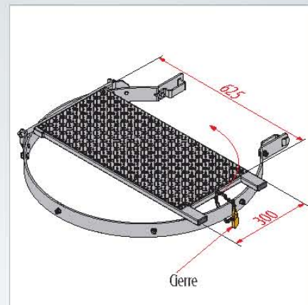
Plataforma intermedia abatible, cerrable
