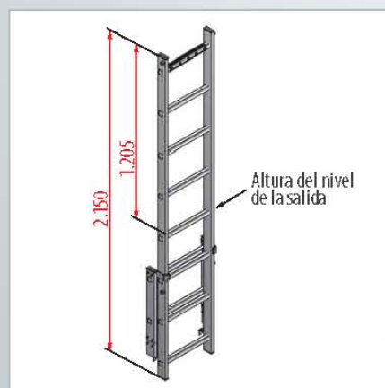
Apoyo de acceso extensible
