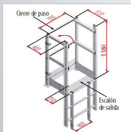
Salida ancha con pasamanos
