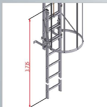
Acceso escamoteable para sistemas confeccionados de escaleras completas
