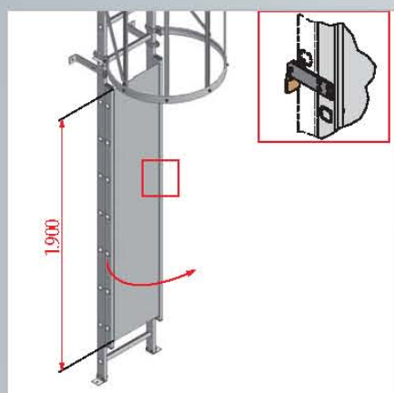
Bloqueo de ascenso, cerrable
