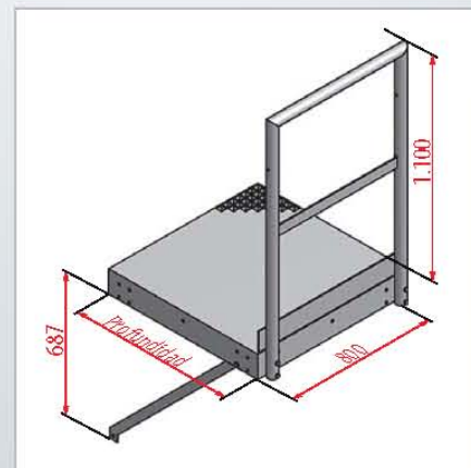
Descansillo complementario pequeño/grande
