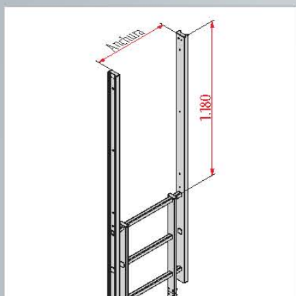
Salida recta, estrecha/ancha
