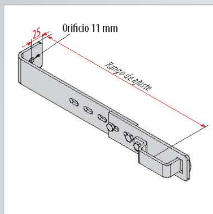
Fijación a la pared ajustable
