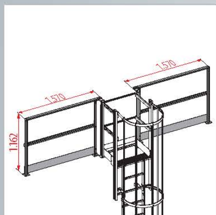
Barandilla para la salida
