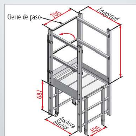
Salida ancha con puente y cierre de paso
