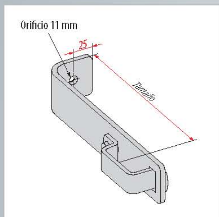
Fijación a la pared estándar
