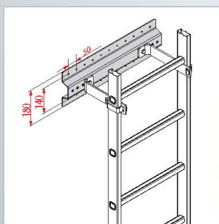
Placa para ganchos de pared en fachadas
