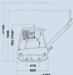
APR 3520 (Honda)
