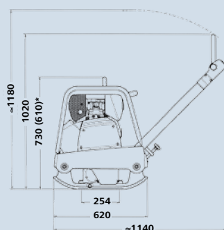
APR 2220 (Honda)
