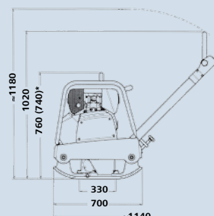
APR 3020 (Honda)
