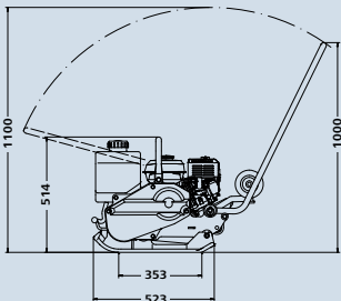
APF 1250 Honda/Subaru
