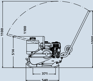
APF 1240 Honda/Subaru
