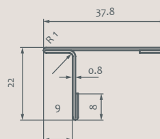
Tapajuntas Premarco Couvre-joints Pré-cadre
