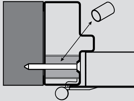
Sistema atornillado tipo "B" (Opcional)
