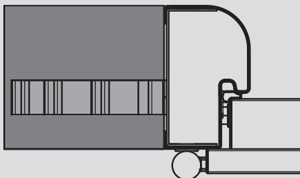
Instalación con garras
