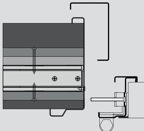
En imagen montado sobre marco CS5
