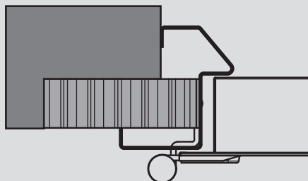
Instalación con garra Ensamblada - Stam - E-Quo - E-Tour - Basic - Office
