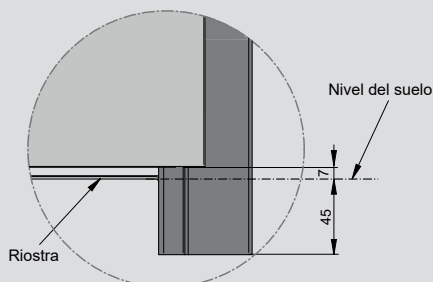
Con pata de cerco
