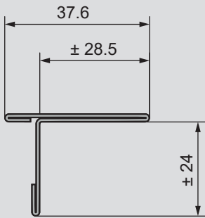
Tapajuntas Premarco
