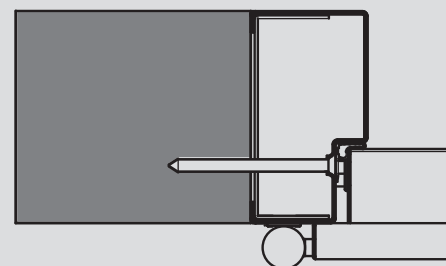
Sistema atornillado
