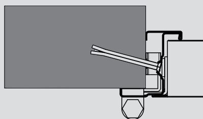
Sistema atornillado oblicuo
