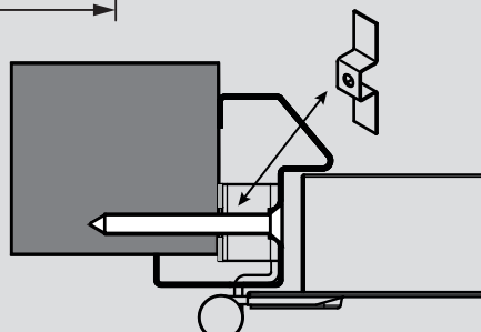
Sistema atornillado Office - E-Quo Opcional: Ensamblada
