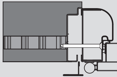
Sistema montaje a Premarco
