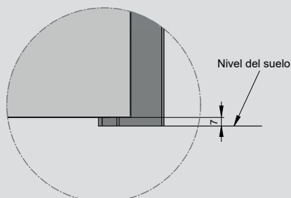
Sin pata de cerco
