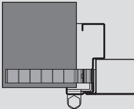
Instalación con garra
