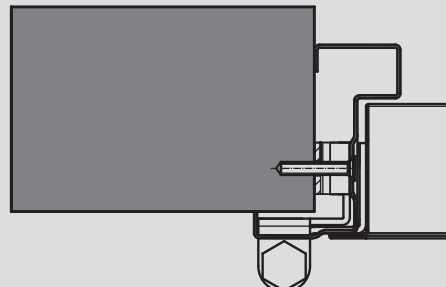
Sistema atornillado
