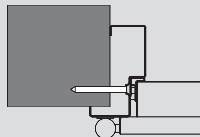
Sistema atornillado
