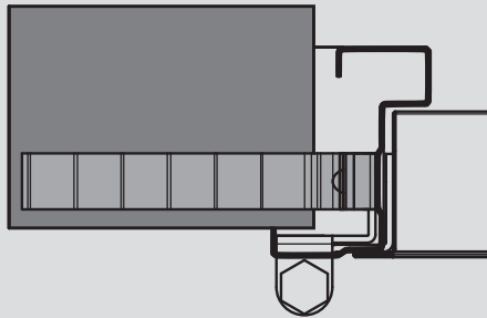
Instalación con garra
