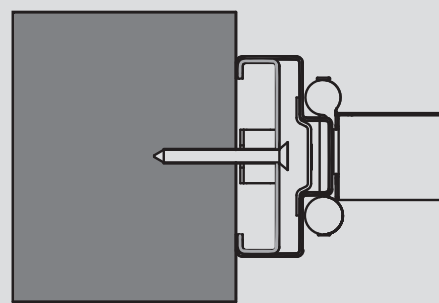
Sistema atornillado
