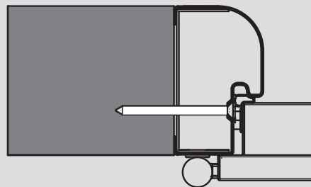
Sistema atornillado
