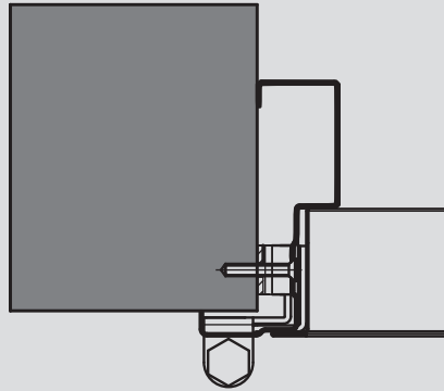
Sistema atornillado
