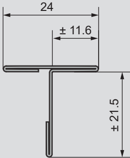
Tapajuntas Fijo
