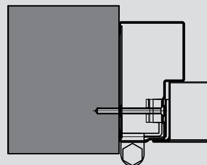
Sistema atornillado
