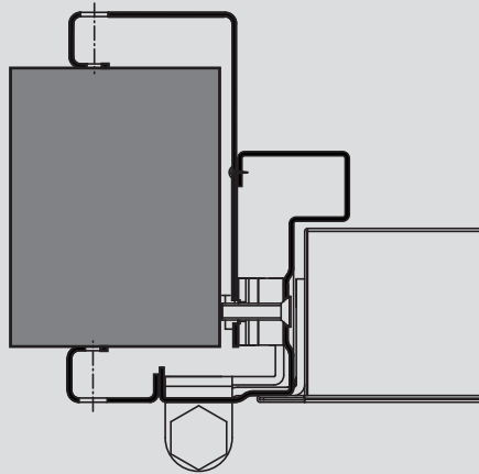
Ala
