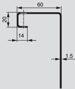
Acople abrazapaneles
