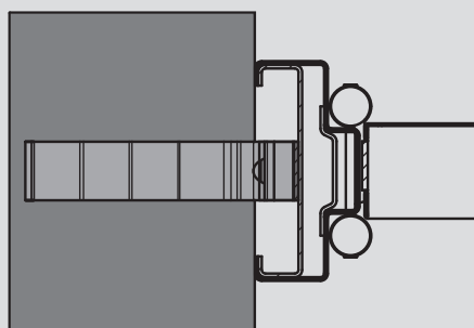
Instalación con garra
