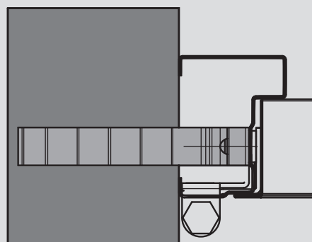
Instalación con garra
