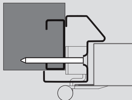
Sistema atornillado tipo "A" (Opcional)
