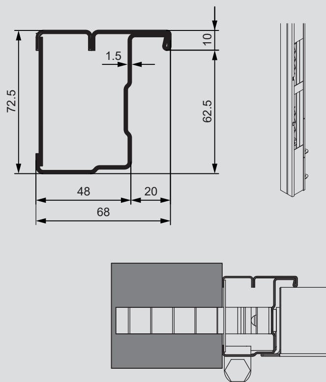
Instalación con garra
