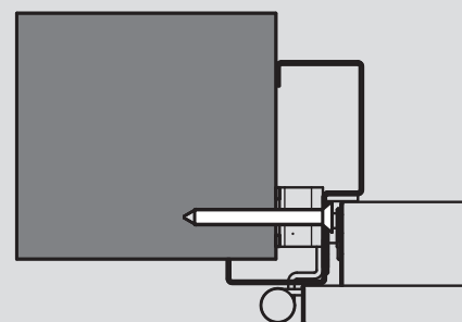
Sistema atornillado (De serie)
