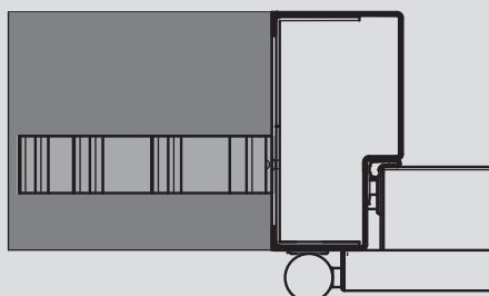
Instalación con garra
