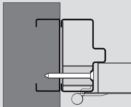
Sistema atornillado tipo "B" (Opcional)
