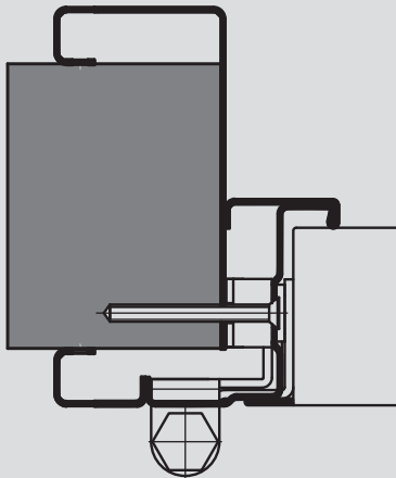
En imagen montado sobre marco CS65
