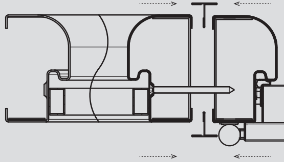
Sistema montaje a Fijo
