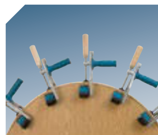
Sujeción de cantos en tableros convexos
