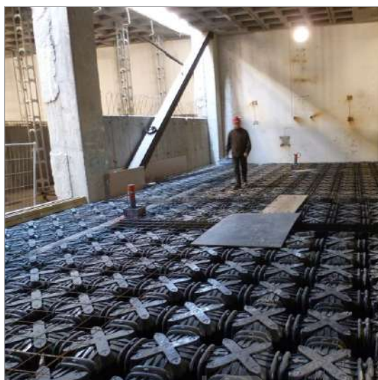
Cámara ventilada para edificio destinado a uso vivienda
