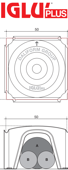
En función de las distintas alturas la forma del encofrado diferirá de la forma en planta.
