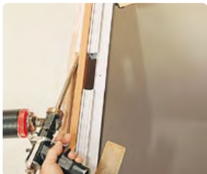
Rellenado con espuma de poliuretano.
