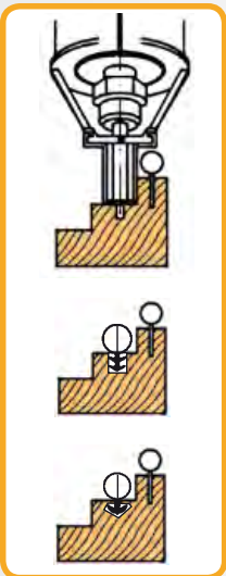
Utilizando la guía recta: ranuras rectas en rebajo de marcos o ventanas.
