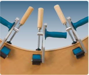
Sujeción de cantos en tableros cóncavos
