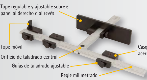
Taladrado para la colocación de estantes.
