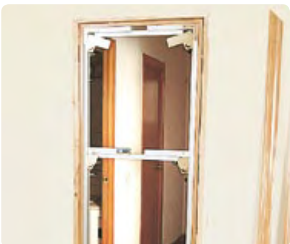
Colocación de la PB83E enrasada con el precerco.
