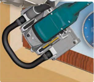
Con el disco de diamante opcional permite un fácil ranurado de las 4 esquinas. Registro por el frontal biselado de la base reversible.
