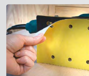
Dos sistemas de sujeción del abrasivo: mediante pinza o velcro (incluido de origen).
