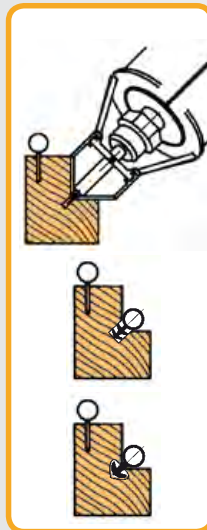
Utilizando la guía de 90°: ranuras oblicuas a 45°, en rebajo de marcos o ventanas.
