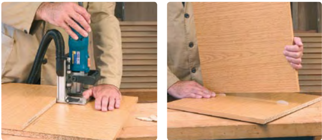
Ensamblaje en medio del tablero
