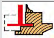
Ranurado de ventana por lado vierte aguas.
