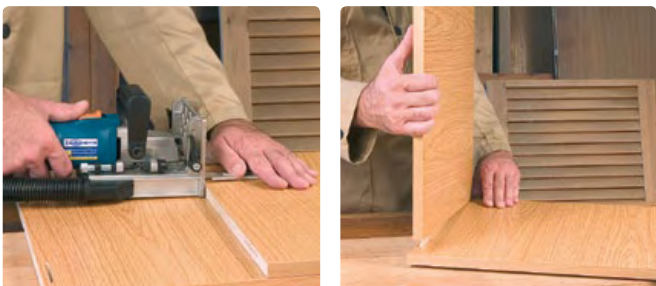
Ensamblaje a escuadra
