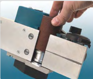
Sustitución de los rodillos lijadores sin herramientas.
