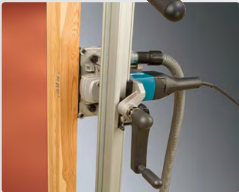
Corte limpio, que permite fijar nuevos cercos directamente en la puerta rehabilitada en un tiempo record y sin esfuerzo.
