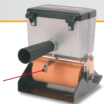
Encolado con el rodillo superior.
