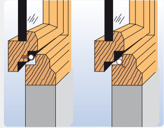
Ranurado en ventanas o puertas y en marcos.
