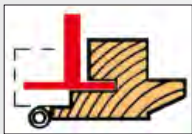
Ranurado de ventana por lado pernios.
