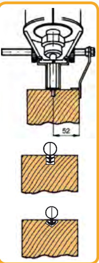
Utilizando la guía recta y la escuadra reversible: ranurar en zonas lisas.
