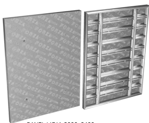
PANEL LIRIA 3000x2400 430 kg/ud. - 7,20 m2/ud.
