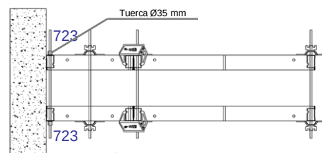
Solución de continuidad en muro en T
