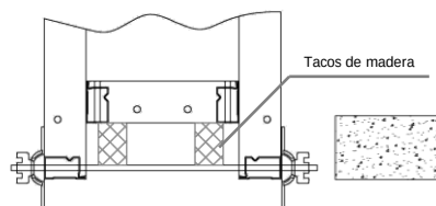
Solución alternativa para los tapes
