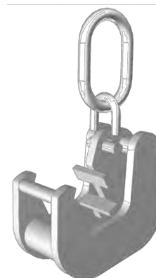
Gancho de elevación 6 kg.
