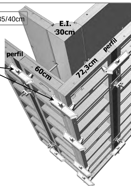
Esquina muro espesor 30cm
