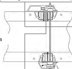
Diwidag a través del marco panel
