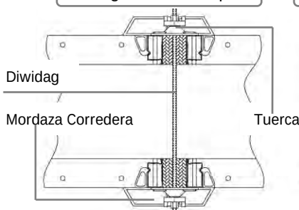
Diwidag a través del perfil
