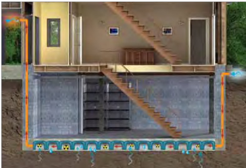
Vivienda construida con unos cimientos ventilados IGLU'®.
