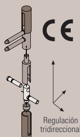
Detalle Bisagra
