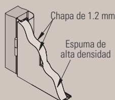
Detalle Relleno
