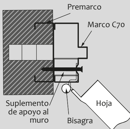
Instalación a marco ancho
