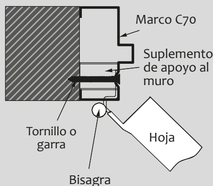
Instalación a premarco
