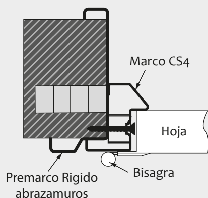
Instalación a premarco abrazamuros
