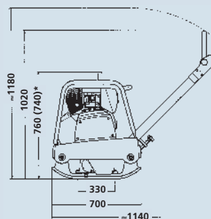
AVP 3020 (*con Honda)
