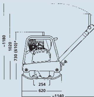
AVP 2220 (*con Honda)
