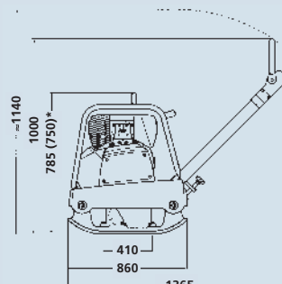
AVP 3520 (*con Honda)
